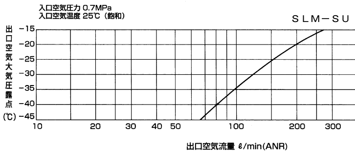
露点性能曲線
